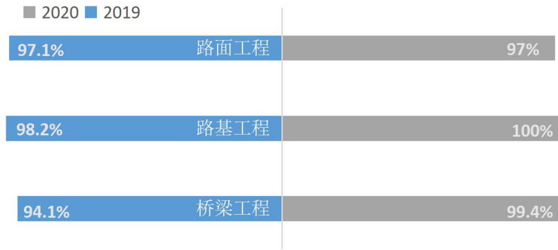
图 1-7 2019、2020 年阜阳市农村公路抽检项目合格率情况
