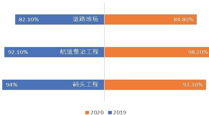
图 1-8 2019、2020 年阜阳市水运工程抽检项目合格率情况
